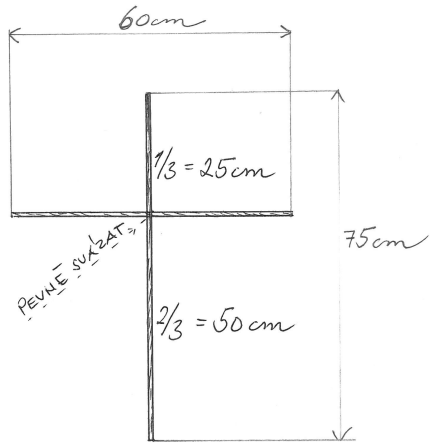
① ROZMĚRY NOSNÍKŮ
