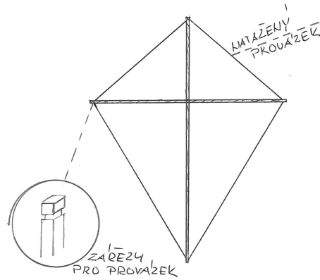
⑤ PŘOTAŽENÍ PŘOUVÁŽKŮ LÍČ
