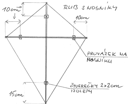
④ PŘOTAŽENÍ PŘOUVÁŽKŮ RUB
