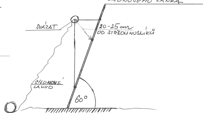
⑥ SKLON PRO UVMÁŽÁNÍ SILNOVÉHO LANKA
